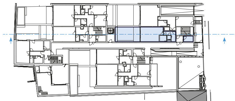
Půdorys 1. NP
