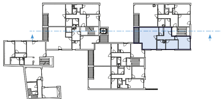
Půdorys 2. NP
