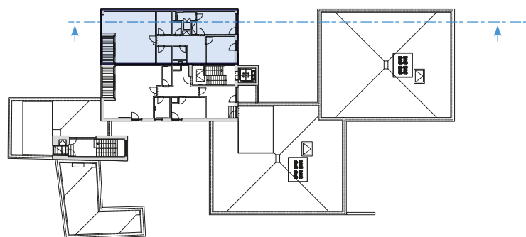
Půdorys 3. NP
